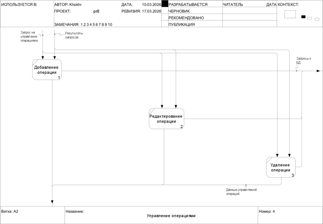
Рисунок 2.9 — Диаграмма DFD. Декомпозиция "Управление операциями"
